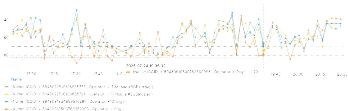
Mierzone RSSI poszczególnych karty
