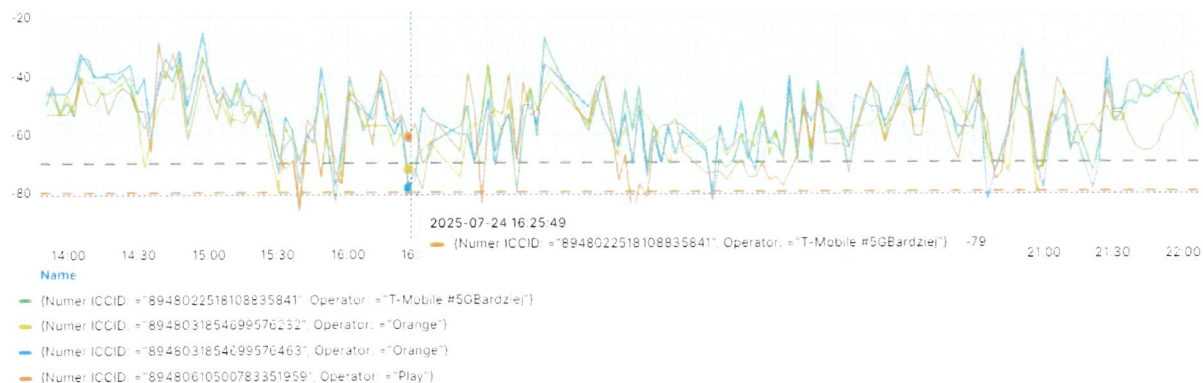
Mierzone RSSI poszczególnej karty
